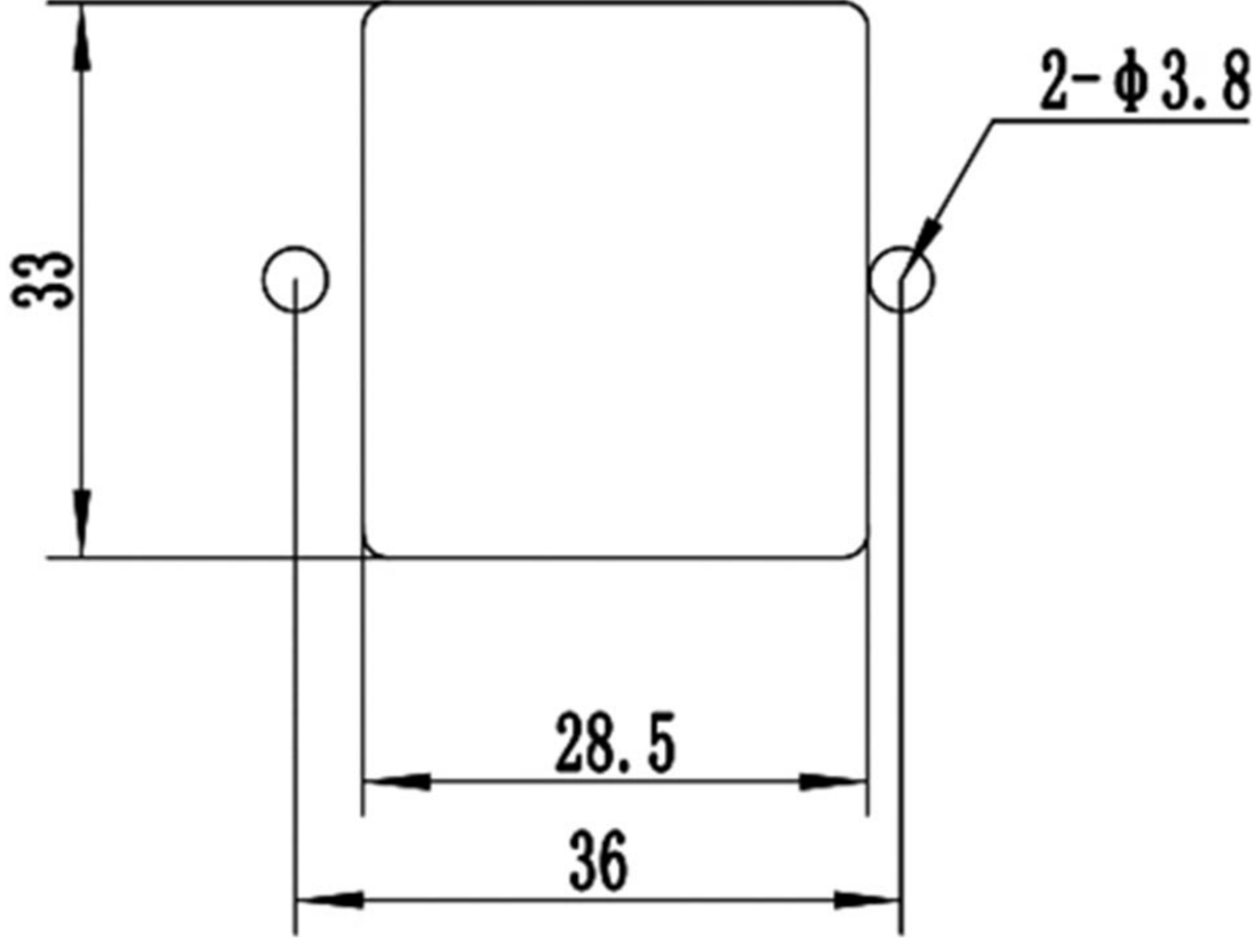
安装尺寸示意图
